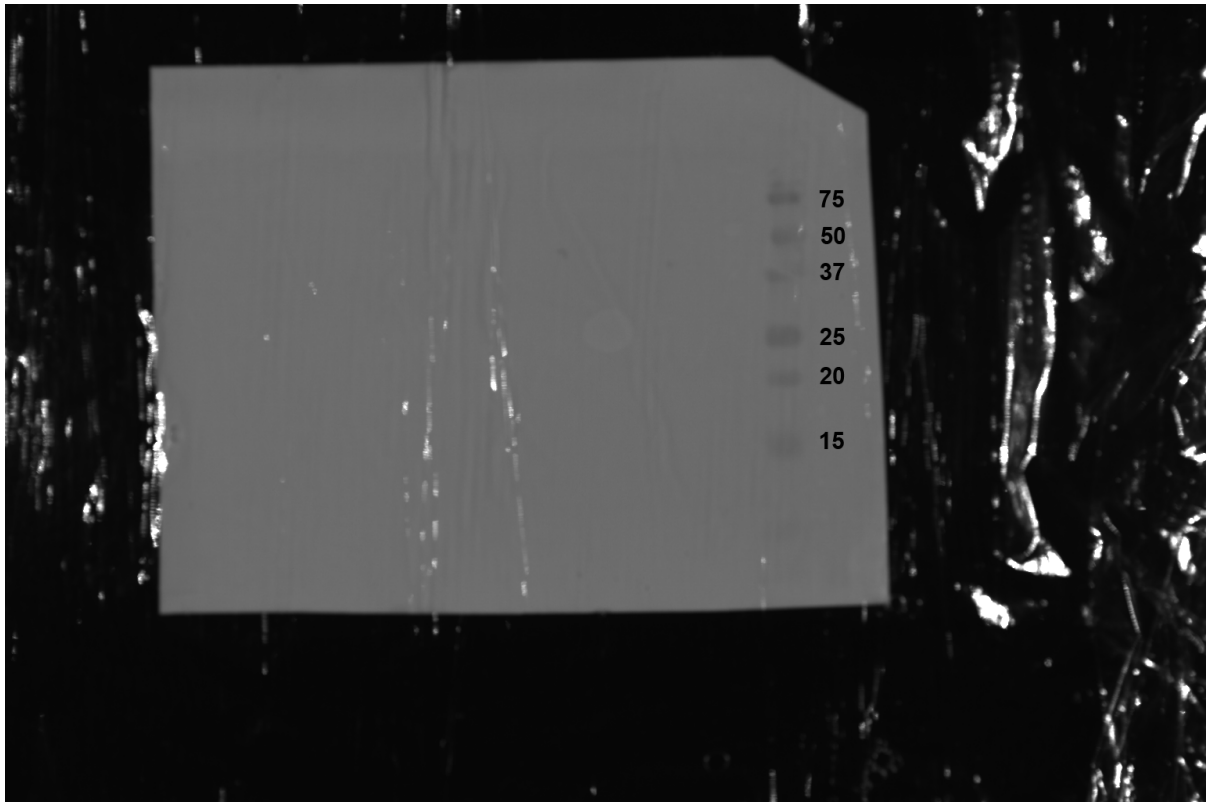
Expression DIG
